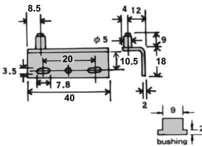
Penture pour porte de bois avec accessoires Wood door hinge with accessories
